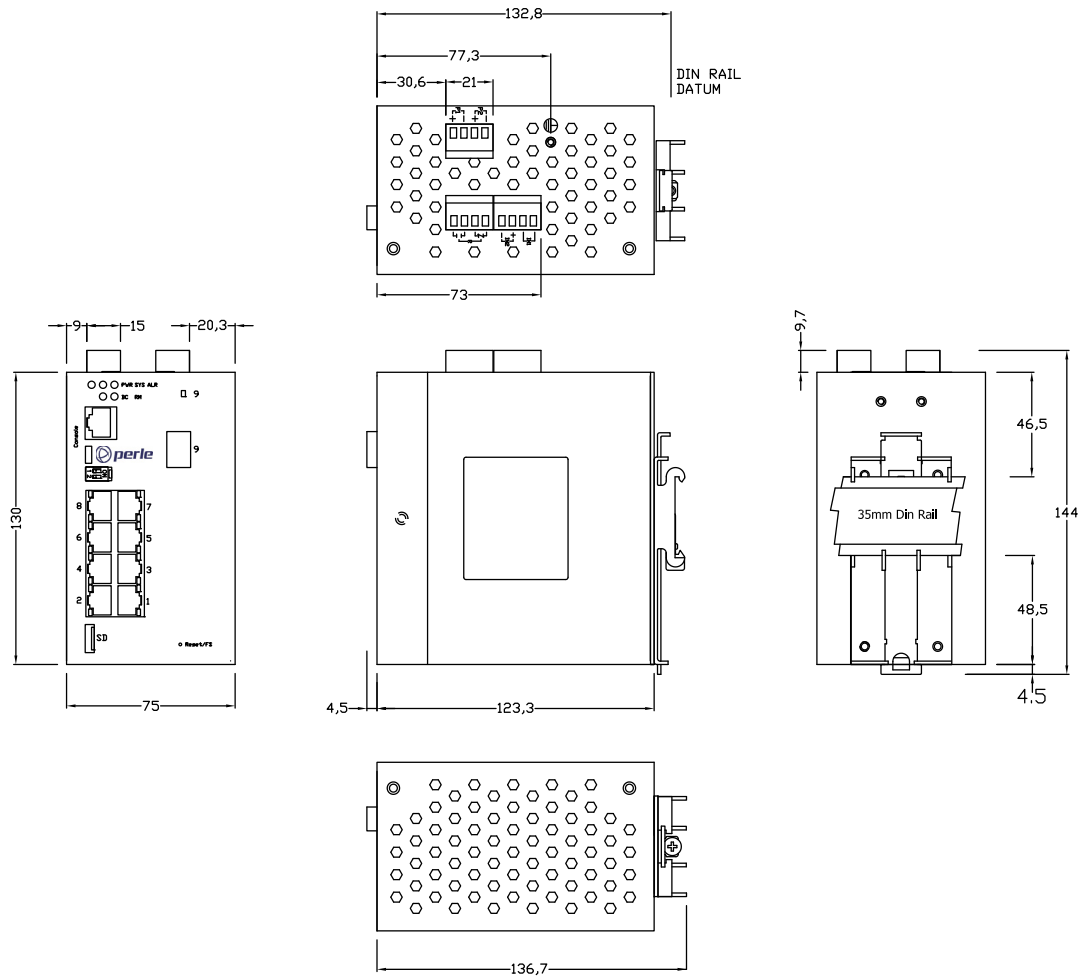
8RJ + 1 SFP
