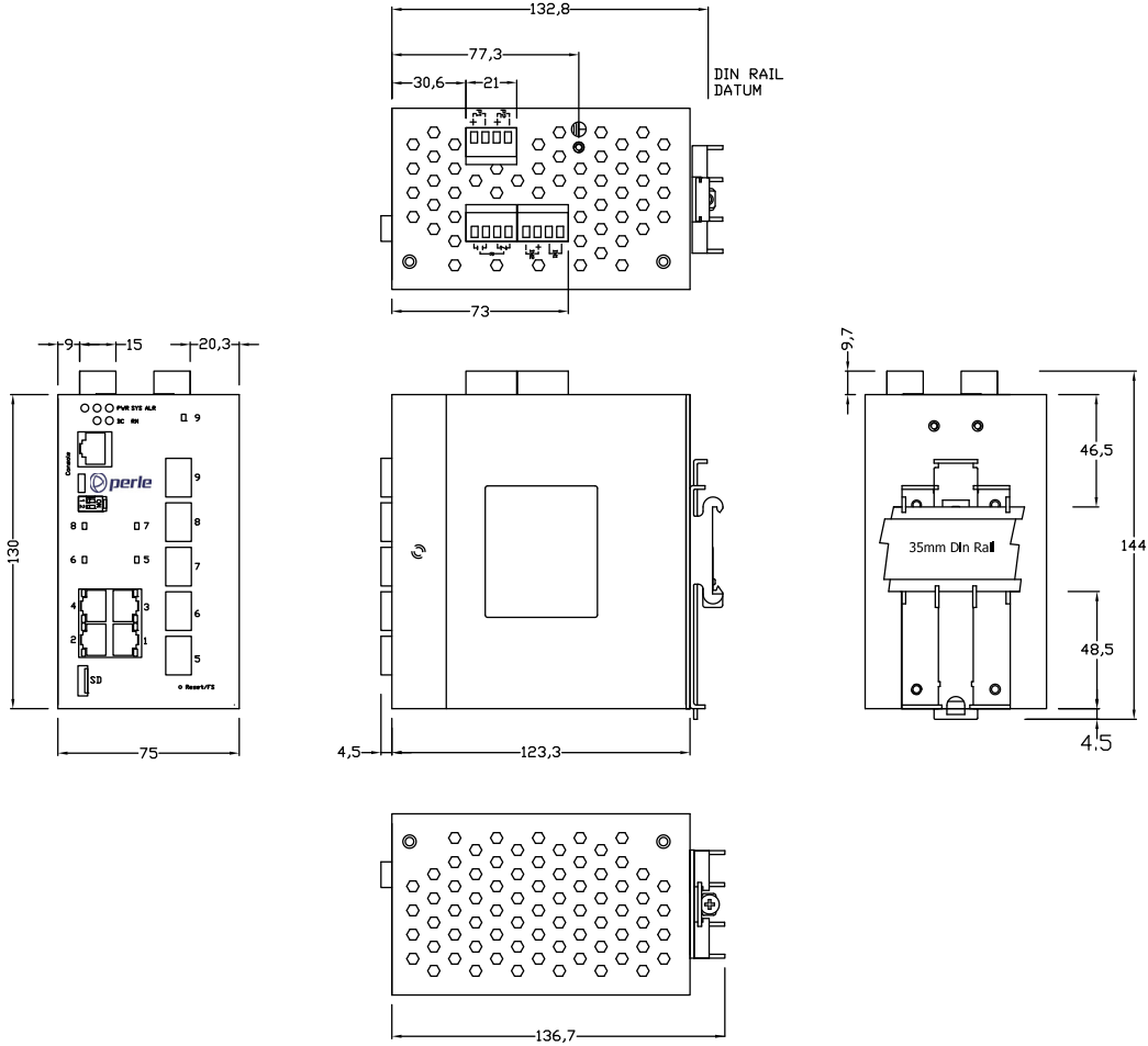
4RJ + 5 SFP
