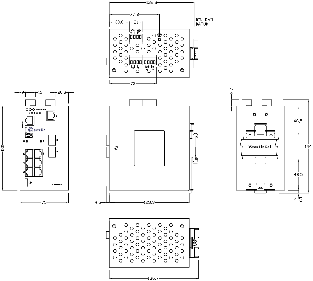
7RJ + 2 SFP
