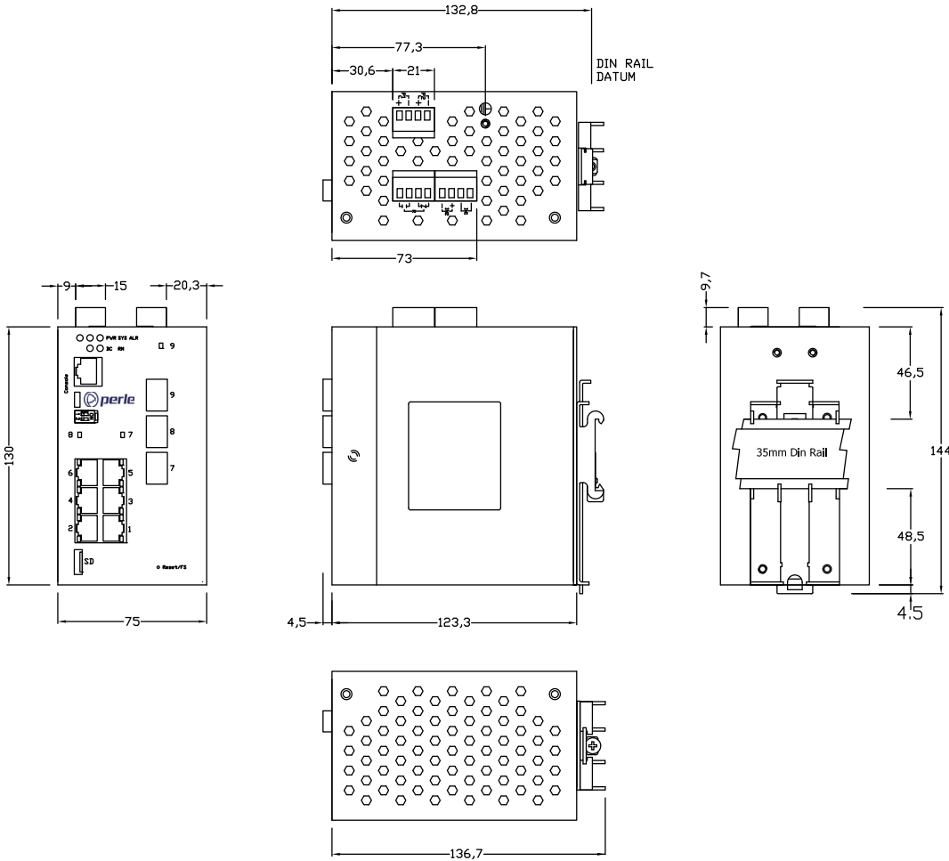
6RJ + 3 SFP
